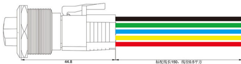
钥匙钮与连接器组合图：
