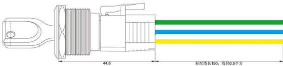
钥匙钮与连接器组合图：
